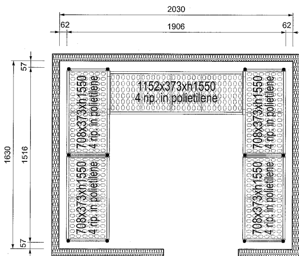
Boven aanzicht
